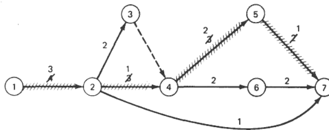
FIGURA 12-18 Intensificación de la ruta crítica.
