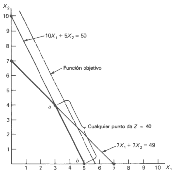
FIGURA 8-3 Ejemplos con soluciones múltiples.
