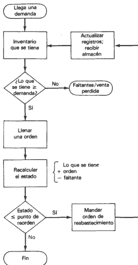
FIGURA 13-2 Modelo de cantidad fija de reorden.
