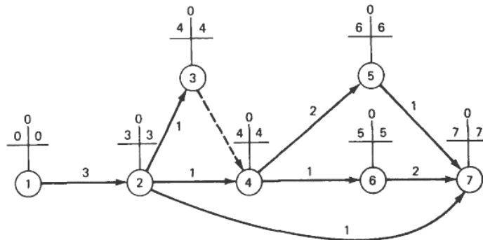
FIGURA 12-19 Red de tiempo mínimo-costo mínimo.
