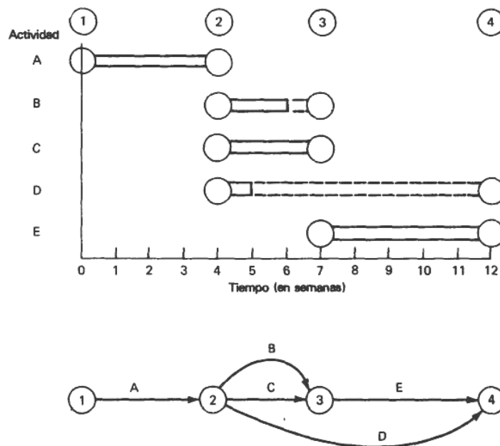
FIGURA 12-2 De la gráfica de Gantt al diagrama de red.
