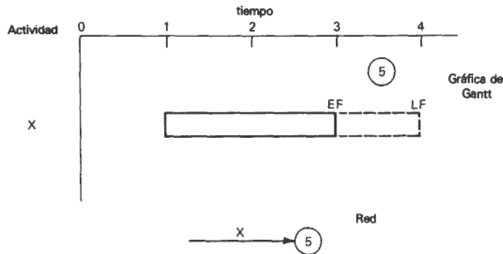
FIGURA 12-6 Tiempos próximo y lejano de un evento.
