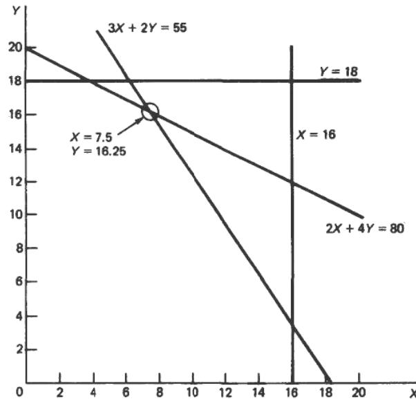
FIGURA 9-4 Ejemplo de programación entera.
