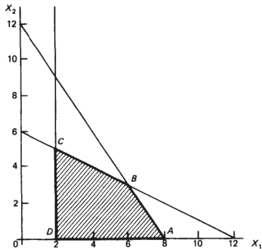
FIGURA 7-7 Frontera extrema de la región factible
