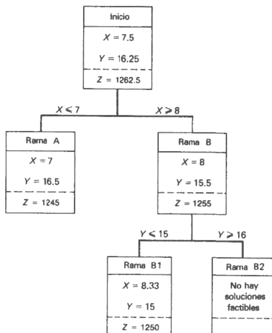
FIGURA 9-8 Traslado a lo largo de la rama B.
