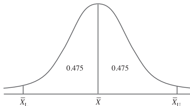
Figura 12.1 Intervalo de confianza del 95 por ciento
