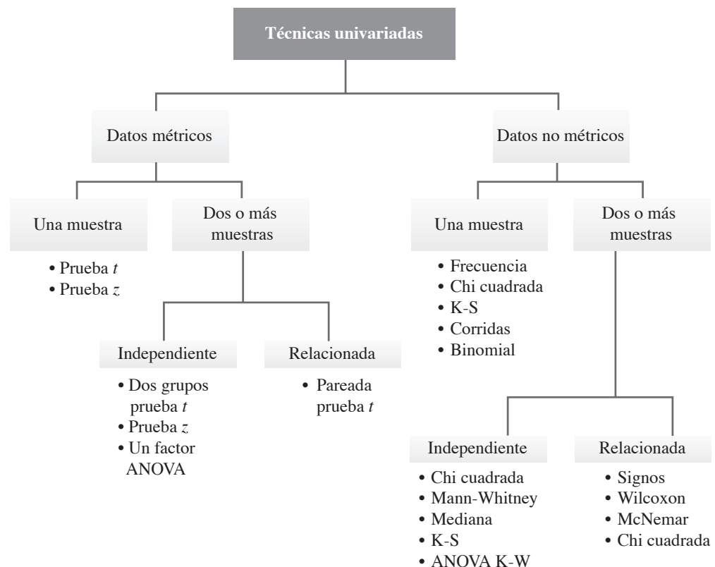
Figura 14.6 Clasificación de las técnicas univariadas
