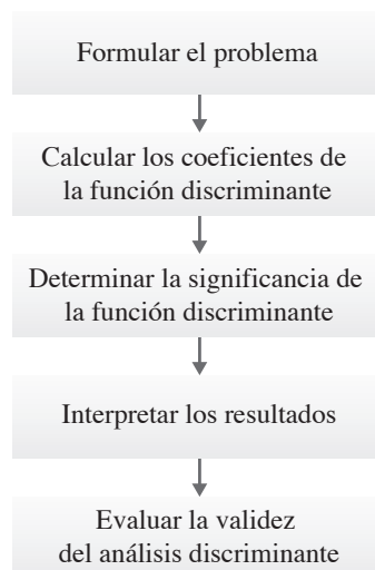
Figura 18.2 Realización de un análisis discriminante
