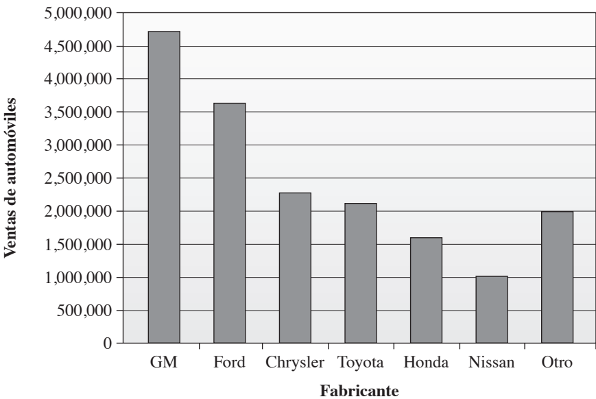
Figura 22.6 Histograma de ventas de automóviles por fabricante (2004)
