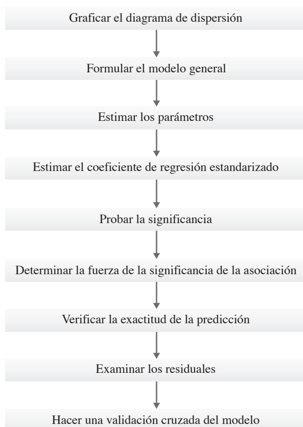
Figura 17.2 Realización del análisis de regresión bivariada
