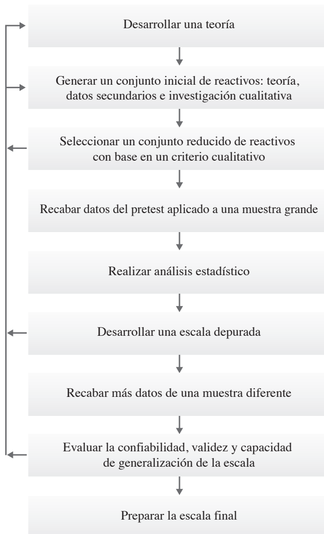
Figura 9.4 Desarrollo de una escala de reactivos múltiples
